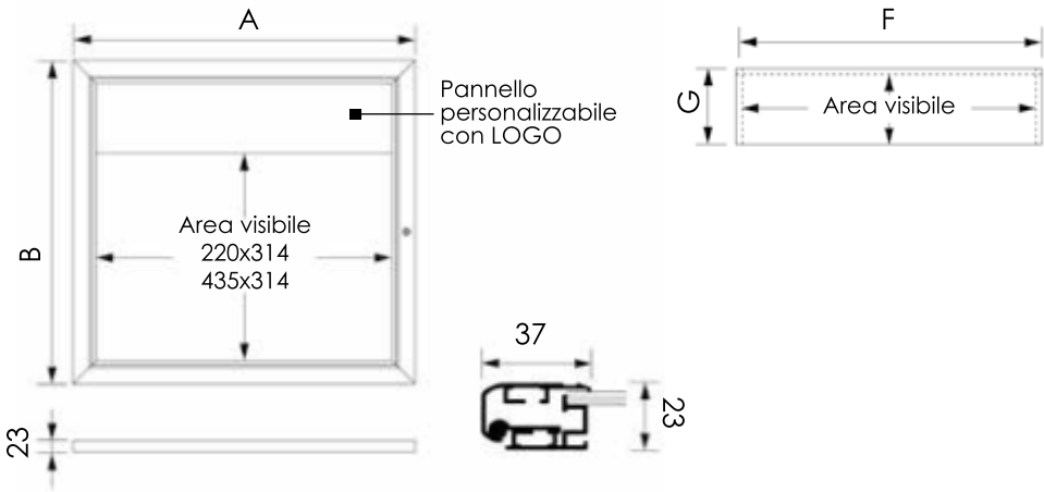
DIMENSIONI CORNICE
