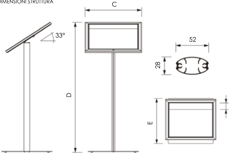
DIMENSIONI STRUTTURA
