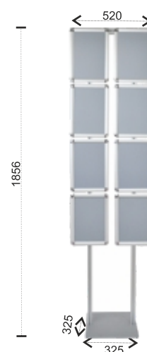
SST-PMA841V SST-PMA842V
