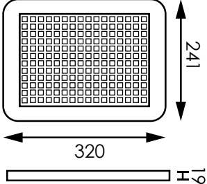
COPERCHIO
