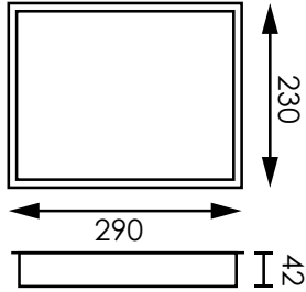
VASCHETTA
