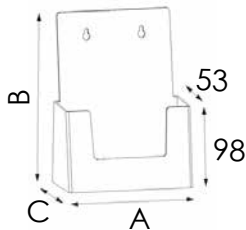
DA5P DIMENSIONE INTERNA SCOMPARTI Larghezza: 153 mm Profondità: 48 mm
