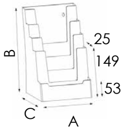
4DA5P DIMENSIONE INTERNA SCOMPARTI Larghezza: 153 mm Profondità: 23 mm
