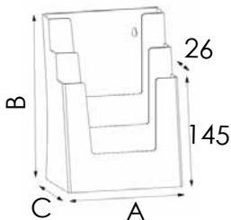
3DA5P DIMENSIONE INTERNA SCOMPARTI Larghezza: 153 mm Profondità: 23 mm
