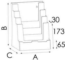
4DA4P DIMENSIONE INTERNA SCOMPARTI Larghezza: 223 mm Profondità: 28,5 mm
