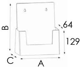
DA4P DIMENSIONE INTERNA SCOMPARTI Larghezza: 222 mm Profondità: 59 mm
