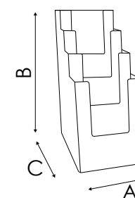
PDB302 DIMENSIONE INTERNA SCOMPARTI Larghezza: 104 mm Profondità: 32 mm
