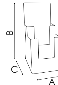
PDB102 DIMENSIONE INTERNA SCOMPARTI Larghezza: 110 mm Profondità: 32 mm
