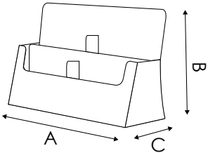
PDR401 DIMENSIONE INTERNA SCOMPARTI Larghezza: 152 mm Profondità: 30 mm
