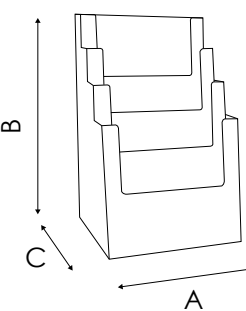
PDB401 DIMENSIONE INTERNA SCOMPARTI Larghezza: 160 mm Profondità: 32 mm
