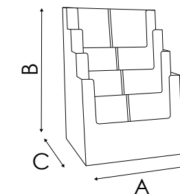
PDB400 DIMENSIONE INTERNA SCOMPARTI Larghezza: 230 mm Profondità: 32 mm
