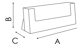
PDB103 DIMENSIONE INTERNA SCOMPARTI Larghezza: 330 mm Profondità: 32 mm
