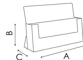
PDB203 DIMENSIONE INTERNA SCOMPARTI Larghezza: 305 mm Profondità: 30 mm
